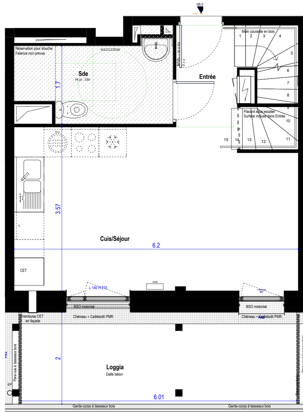
1 2B-2D Bas 1 : 50
